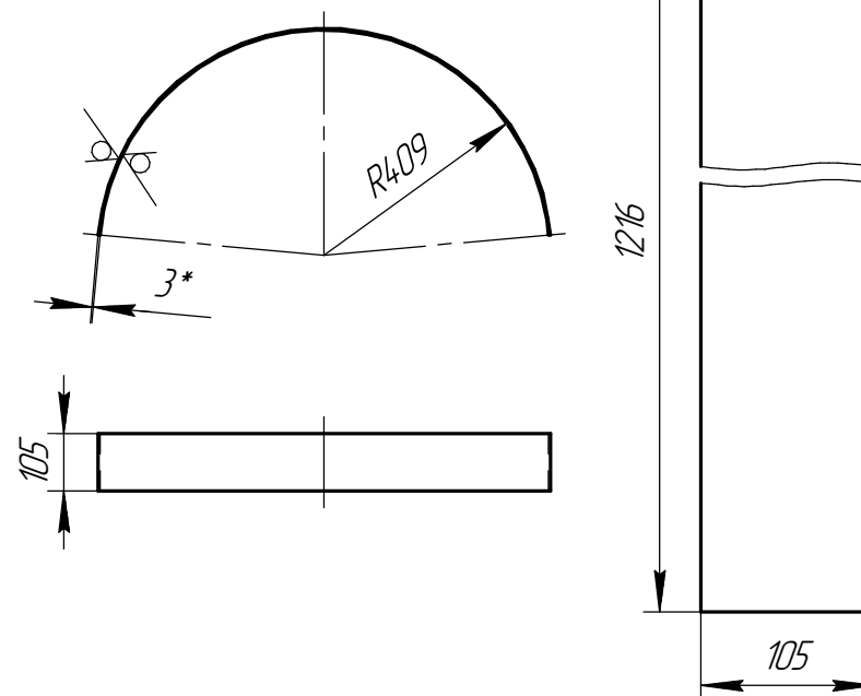
Дет. поз. 8 (1:15)
