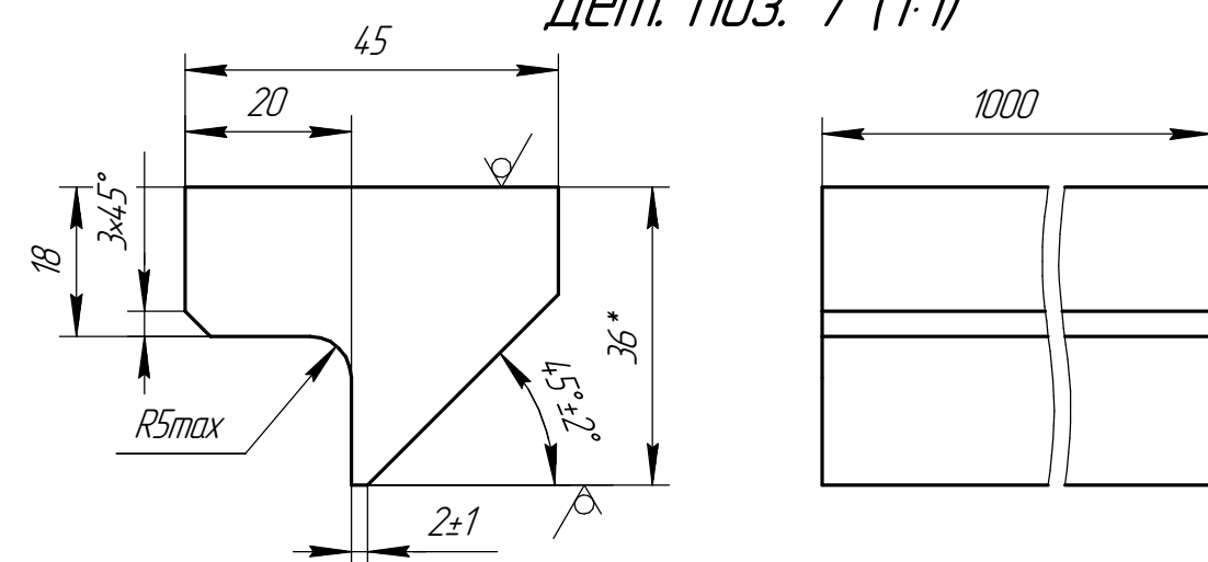
Дет. поз. 7 (1:1)
