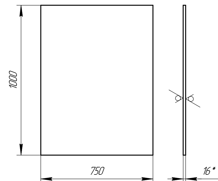
Дет. поз. 6 (1:15)
