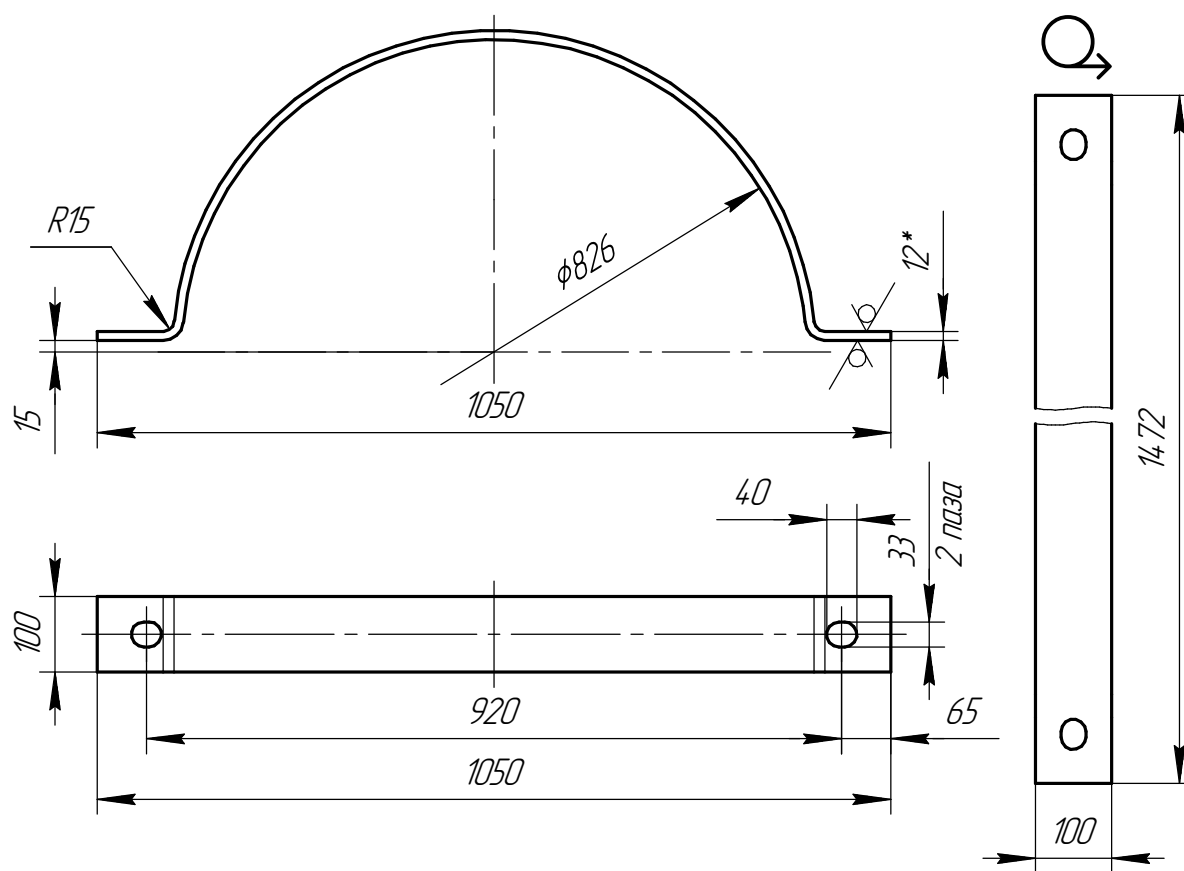
Дет. поз. 7 (1:1)
