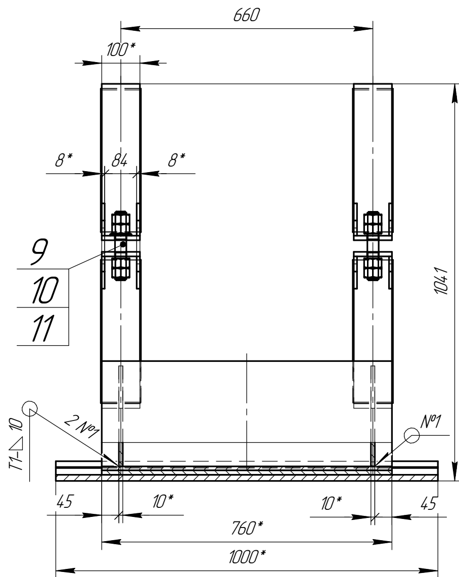
Дет. поз. 3
