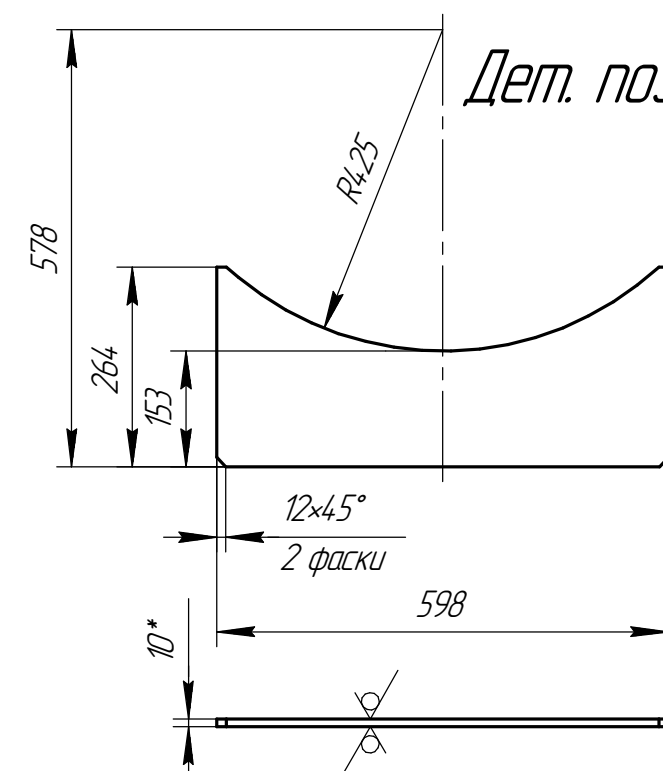
Дет. поз. 6 (1:15)
