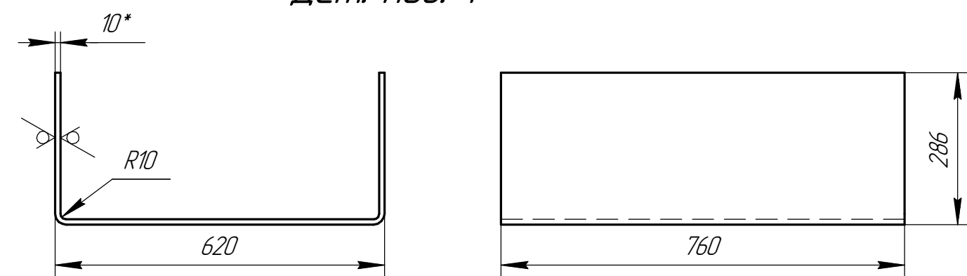
Q (1:15)
